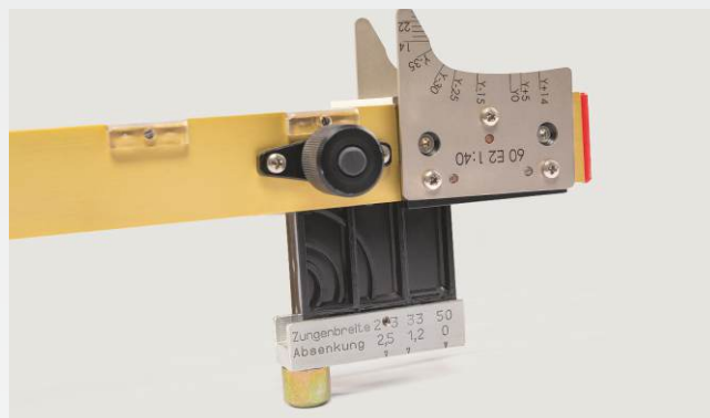
SRQ-Lehre, Kopfbreitenskala (optional)
