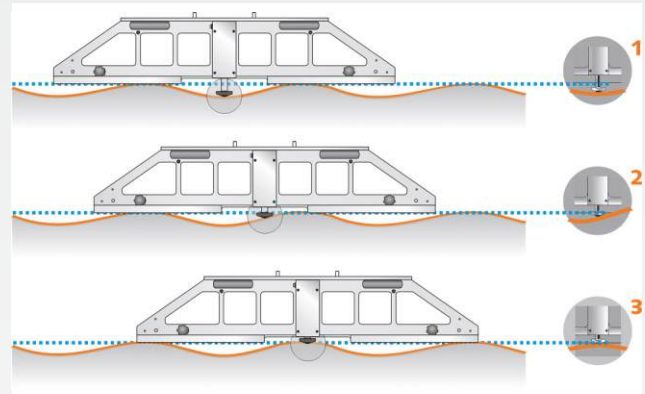
Messprinzip RMF 1100
