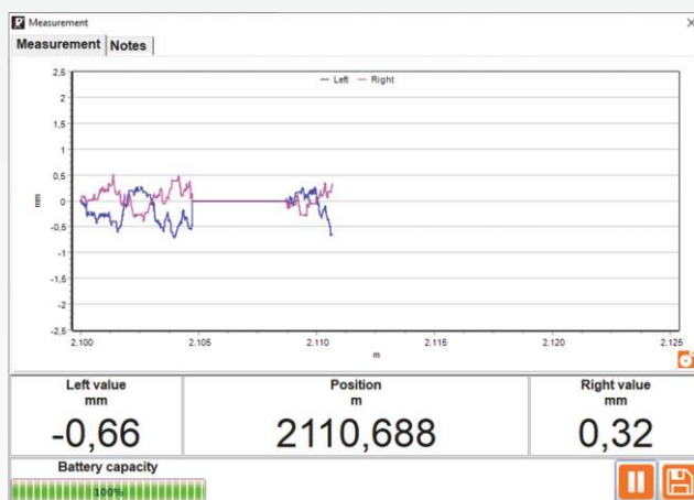
Logiciel de saisie des données RMFcatcher (se mettant en pause)
