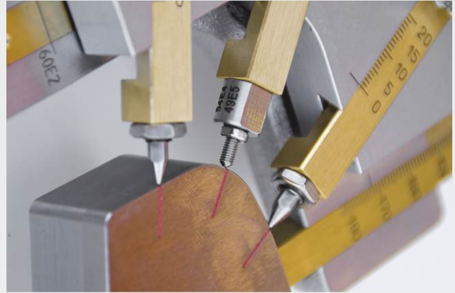
SKM 2: Mesure de l'usure des bords de roulement sur trois points
